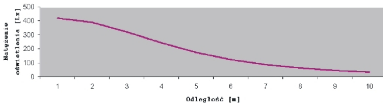
Natężenie oświetlenia wokół lampy HTI 1000
